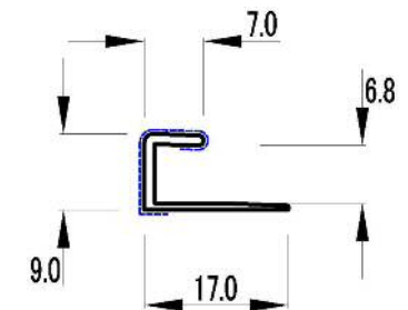
SKエンド見切り -6
