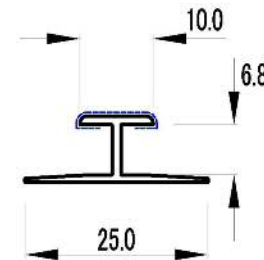
SKジョイナーエ型 -6
